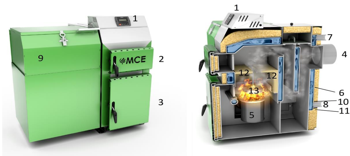
RYS. 1. PRZEKRÓJ KOTŁA V6 8
