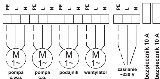
Rys.3 Schemat elektryczny podłączenia przewodów zasilających
