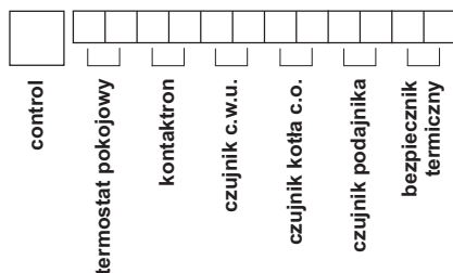
Rys.4 Schemat elektryczny podłączenia czujników
