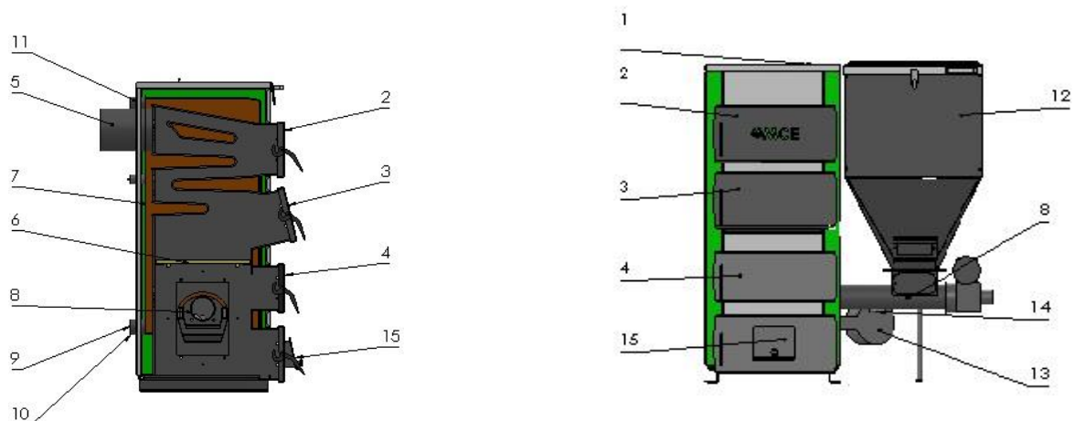
RYS. 1 Przekrój kotła V4
