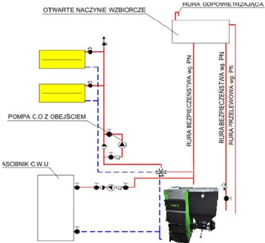
RYS. 2. SCHEMAT INSTALACJI KOTŁA W UKŁADZIE OTWARTYM ZGODNIE Z ISTNIEJĄCYMI PRZEPISAMI.
