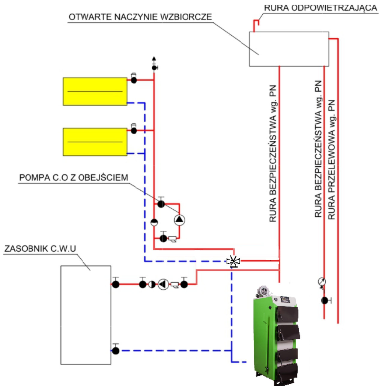
RYS. 3. Schemat montażu kotła z zastosowaniem zaworu czterodrogowego
