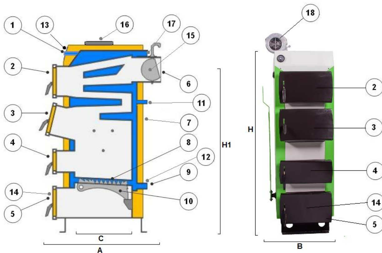
Rys nr 1. Przekrój kotła V2S
