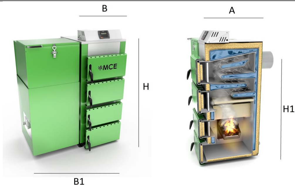
RYS. 2 Wymiary kotła V4
