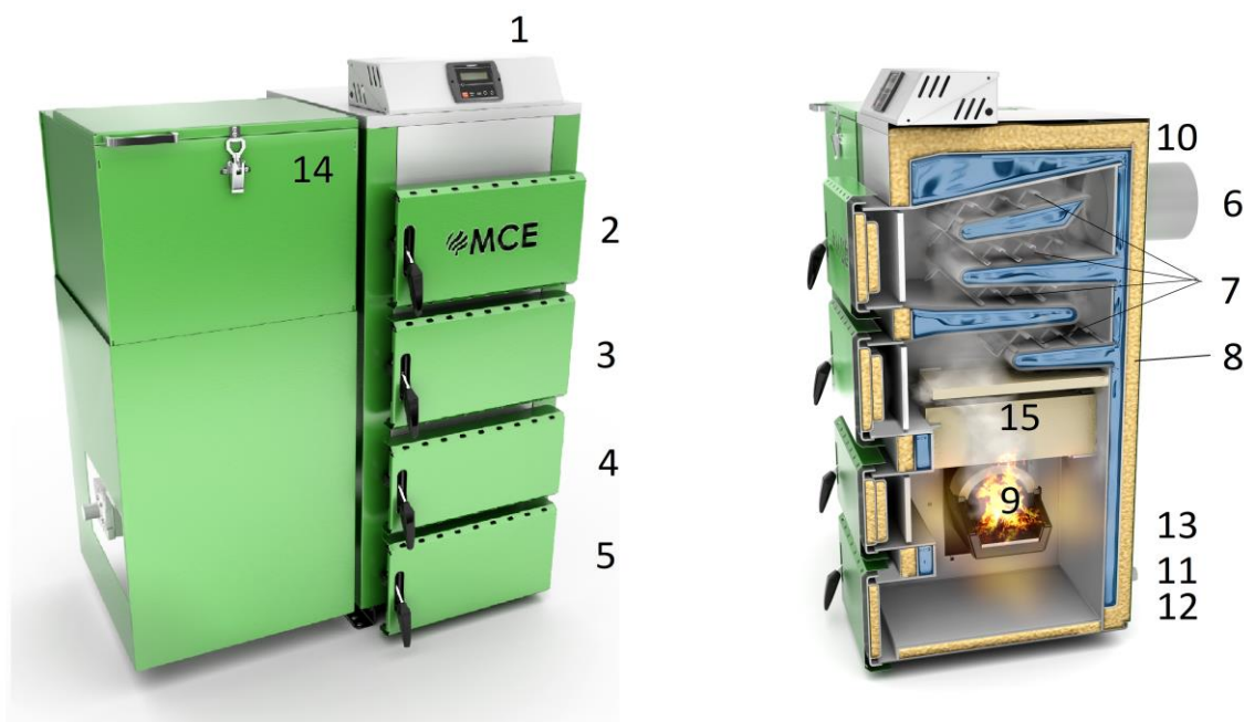
RYS. 1 Przekrój kotła V4
