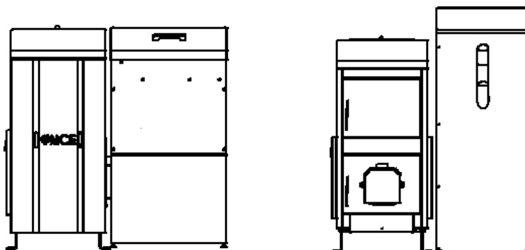
RYS. 2. SPOSOBY MONTAŻU PALNIKA W KOTLE V7 15 KW – Z BOKU KOTŁA (RYS. Z LEWEJ) ORAZ W DRZWICZKACH KOTŁA (RYS. Z PRAWYJ STRONY).
