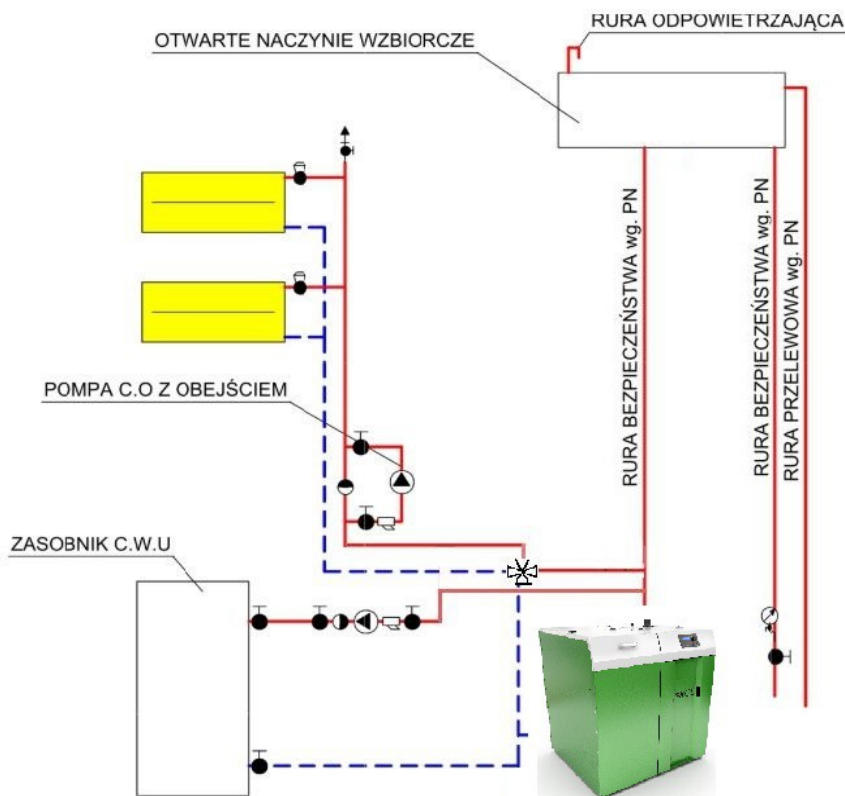
RYS. 2. SCHEMAT INSTALACJI KOTŁA W UKŁADZIE OTWARTYM ZGODNIE Z ISTNIEJĄCYMI PRZEPISAMI.
