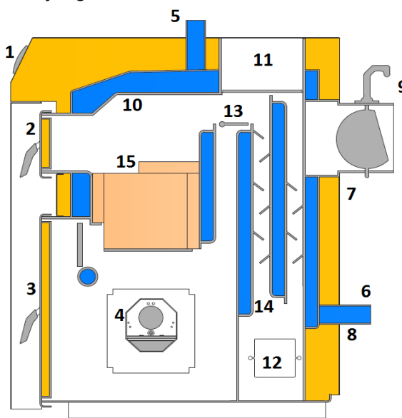
RYS. 1. PRZEKRÓJ KOTŁA V6
