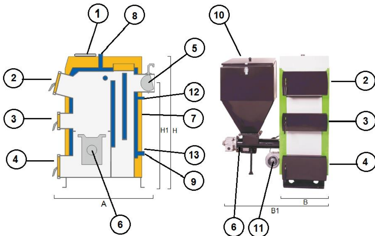
RYS. 1. PRZEKRÓJ KOTŁA V6
