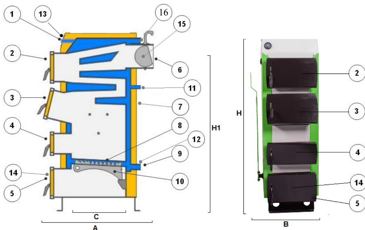
Rys nr 1. Przekrój kotła V2
